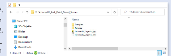
Bild 1: Inhalt
