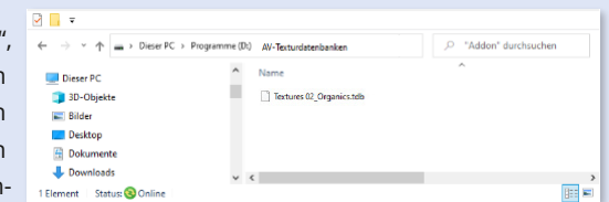
Bild 3: Ordnerinhalt AV-Texturdatenbanken
