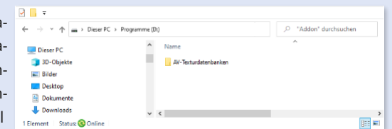
Bild 2: Datenbankordner erstellen
